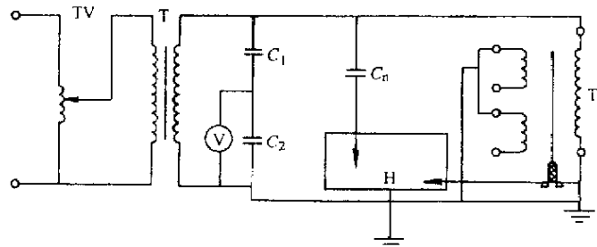
TV——调压器；V——峰值电压表；T——试验变压器；H——电桥； T i ——被试互感器；C n ——标准电容器；C 1 、C 2 ——电容分压器。
