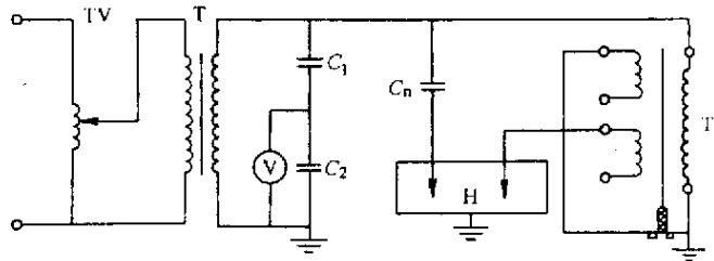
TV——调压器；V——峰值电压表；T——试验变压器；H——电桥； T i ——被试互感器；C n ——标准电容器；C 1 、C 2 ——电容分压器。
