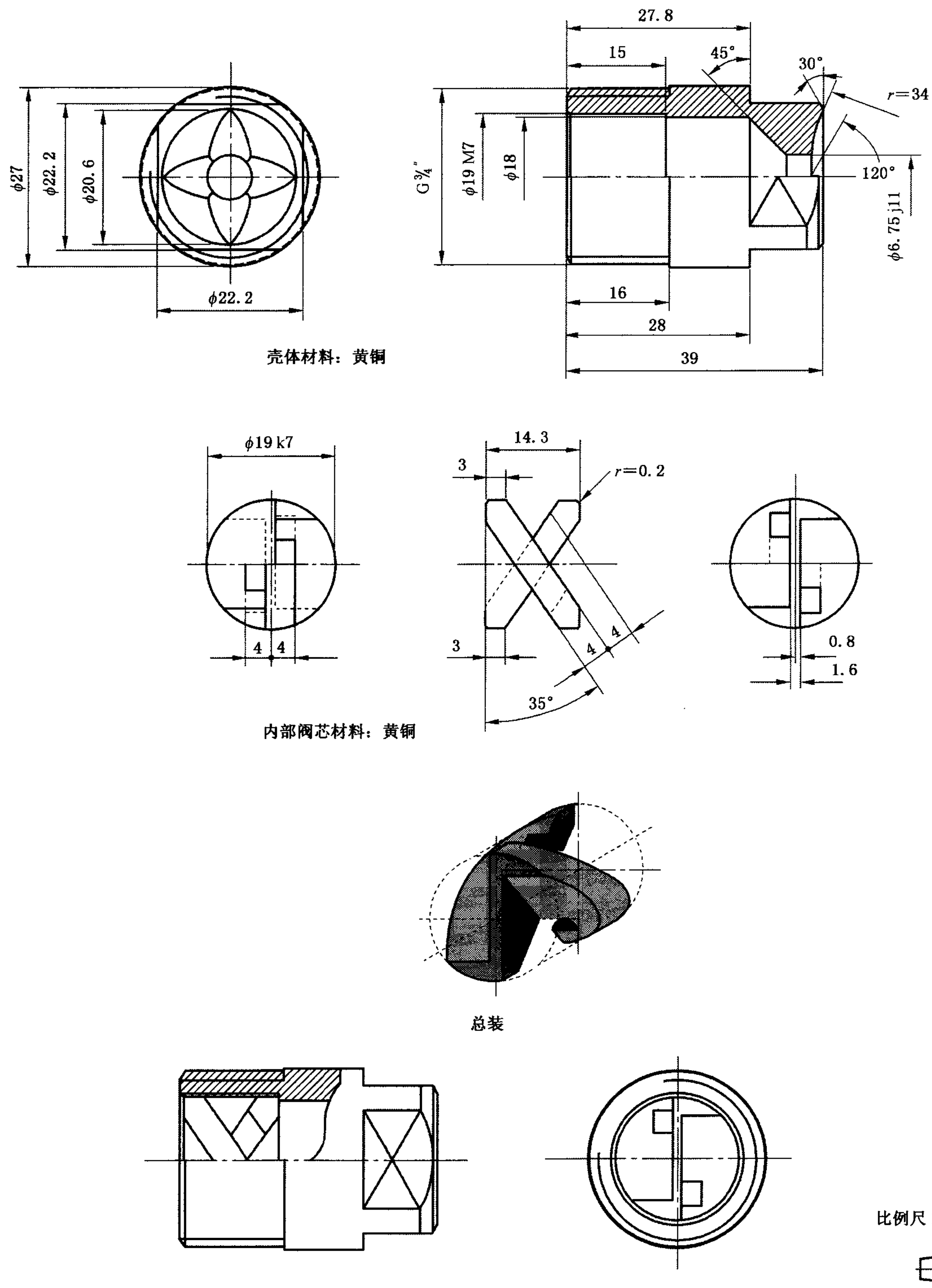
图 C.2 气候防护试验用的喷嘴
